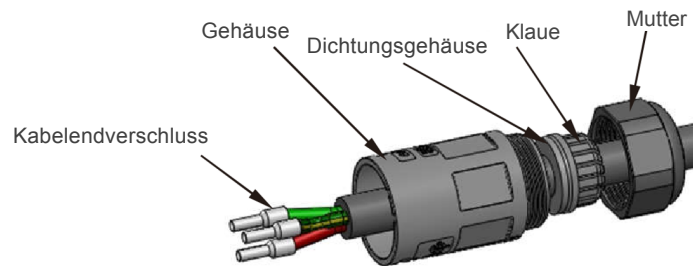
Abbildung 4.14 AC-Netzanschlussklemme
